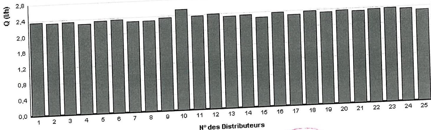
Test d'Homogénéité de fabrication du goutteur NAVIA AUTOREGULANT 2,2 l/h
